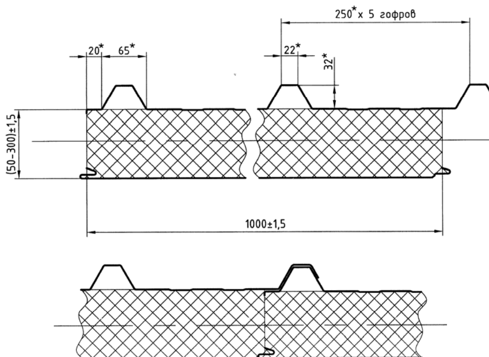
Рис.1. Форма поперечного сечения и размеры панелей
