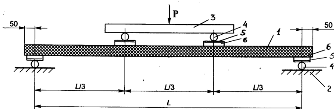
1 - образец; 2 - база; 3 - траверса; 4 - стальные цилиндрические опоры; 5 - стальные пластины; 6 - прокладки
