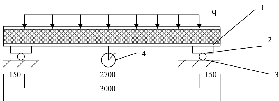
1 – образец; 2 – стальные пластины сечением 100x3 мм; 3 – стальные цилиндрические опоры диаметром 40-50 мм; 4 – прибор для измерения деформаций
